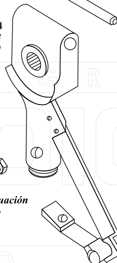
060074 Horquilla Modelo 60 (AT)
