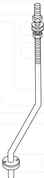
060220 Tornillo P/Tensar el Motor Modelo 60 (AT)
